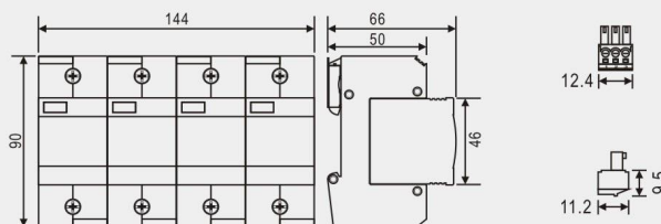
BT P BCM 25 RM/4P Diagrama de dimensiones
