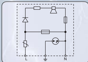
BT E230_Diagrama Circuito Básico
