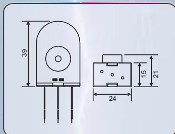
BT E 230 / 230C_Dimensión del Diagrama
